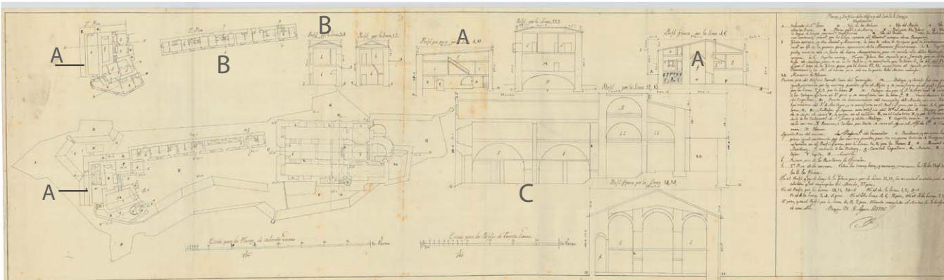
Plànol on es pot apreciar el conjunt del castell i els seus edificis, casa del governador, edifici d'oficials i església. (signat per Josep Gabriel el 1796)
