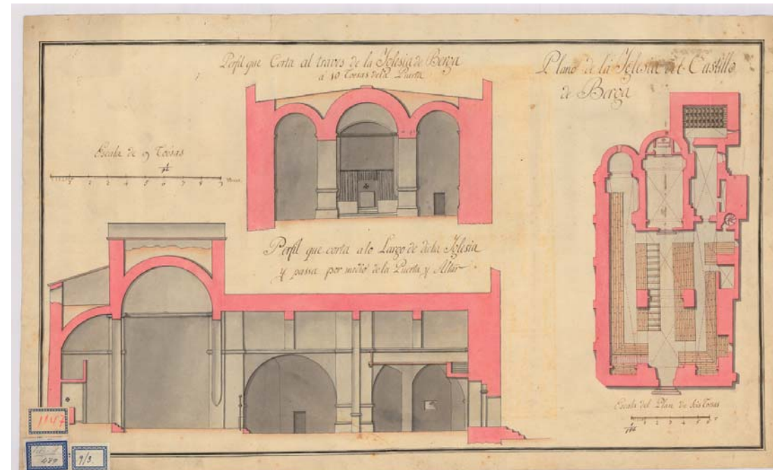
Plànol de l'esglèsia a finals del XVIII
