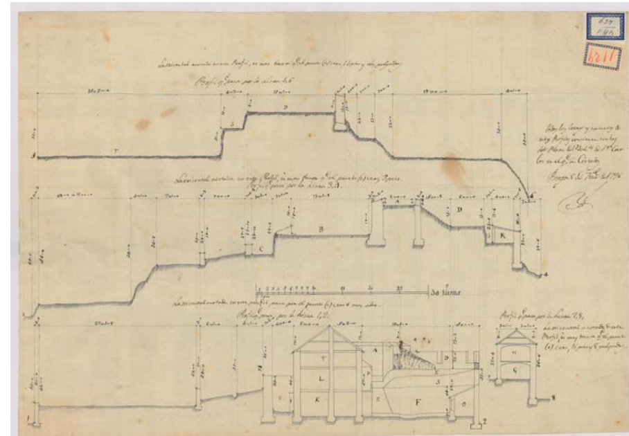
Plànol del 1796 signat per Josep Gabriel on es veuen els perfils i seccions del Baluard de Sant Carles
